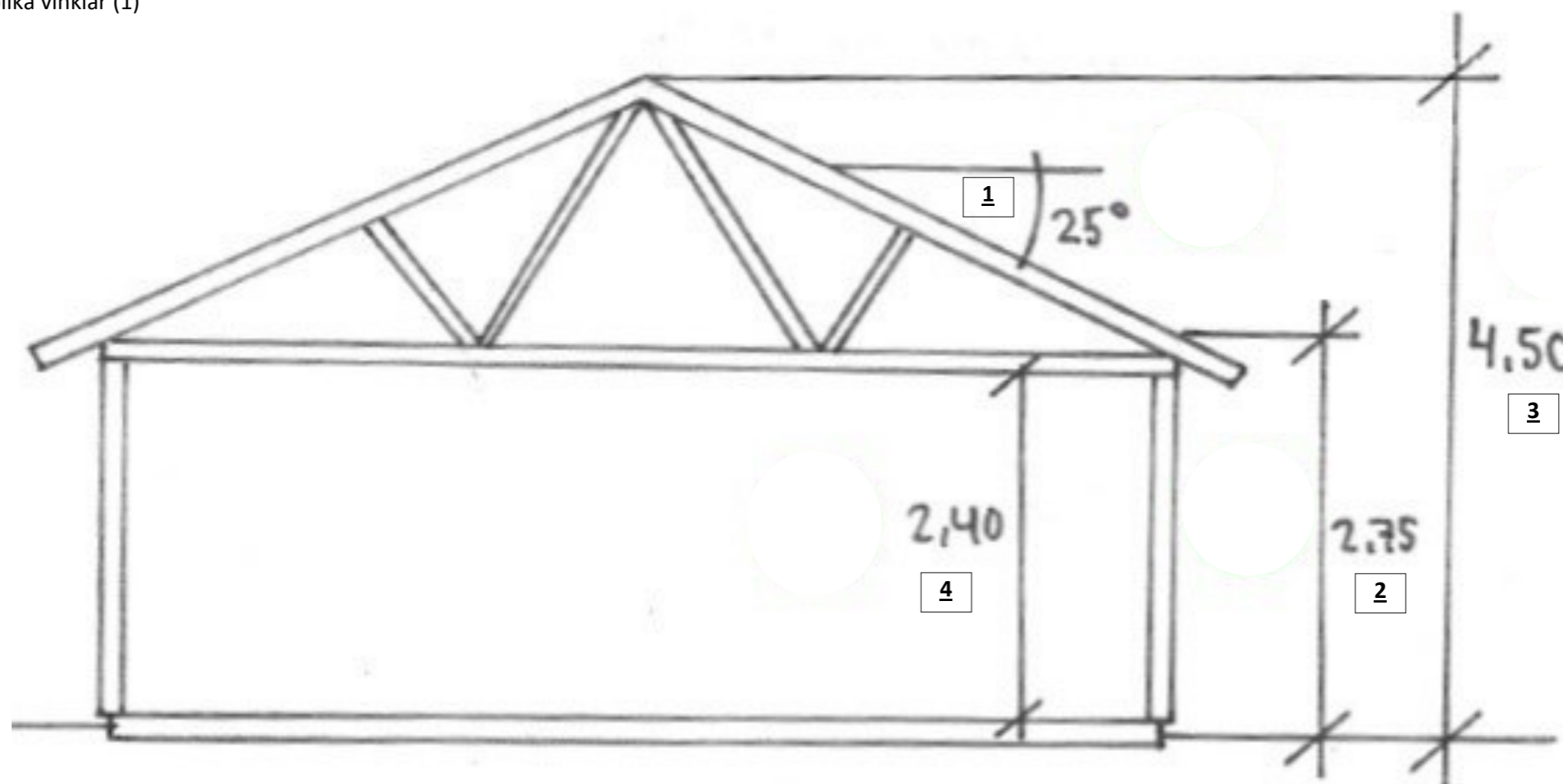
Sektion A-A
